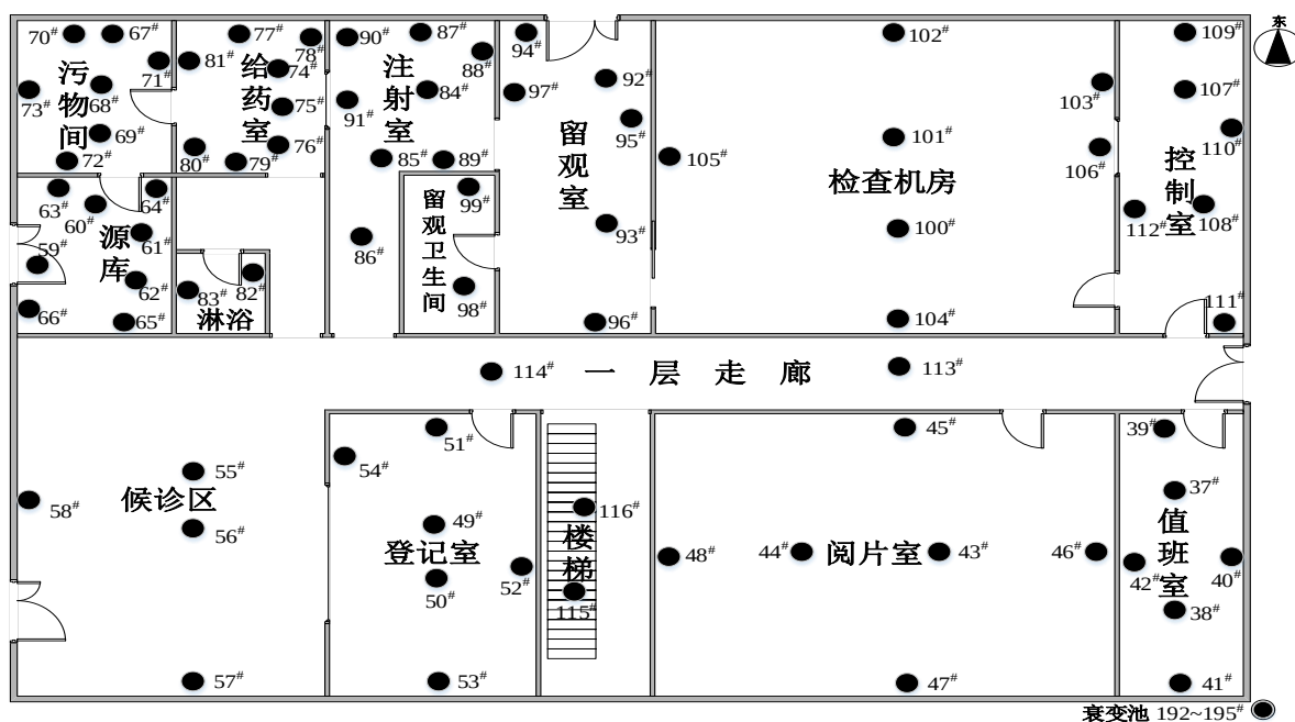
图 4.4 退役核医学科楼一层 \beta 表面污染的检测布点
