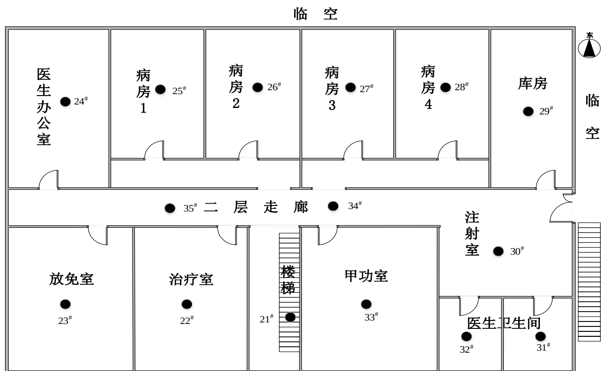
图 4.1 退役核医学科楼二层 \gamma 辐射剂量率的检测布点
