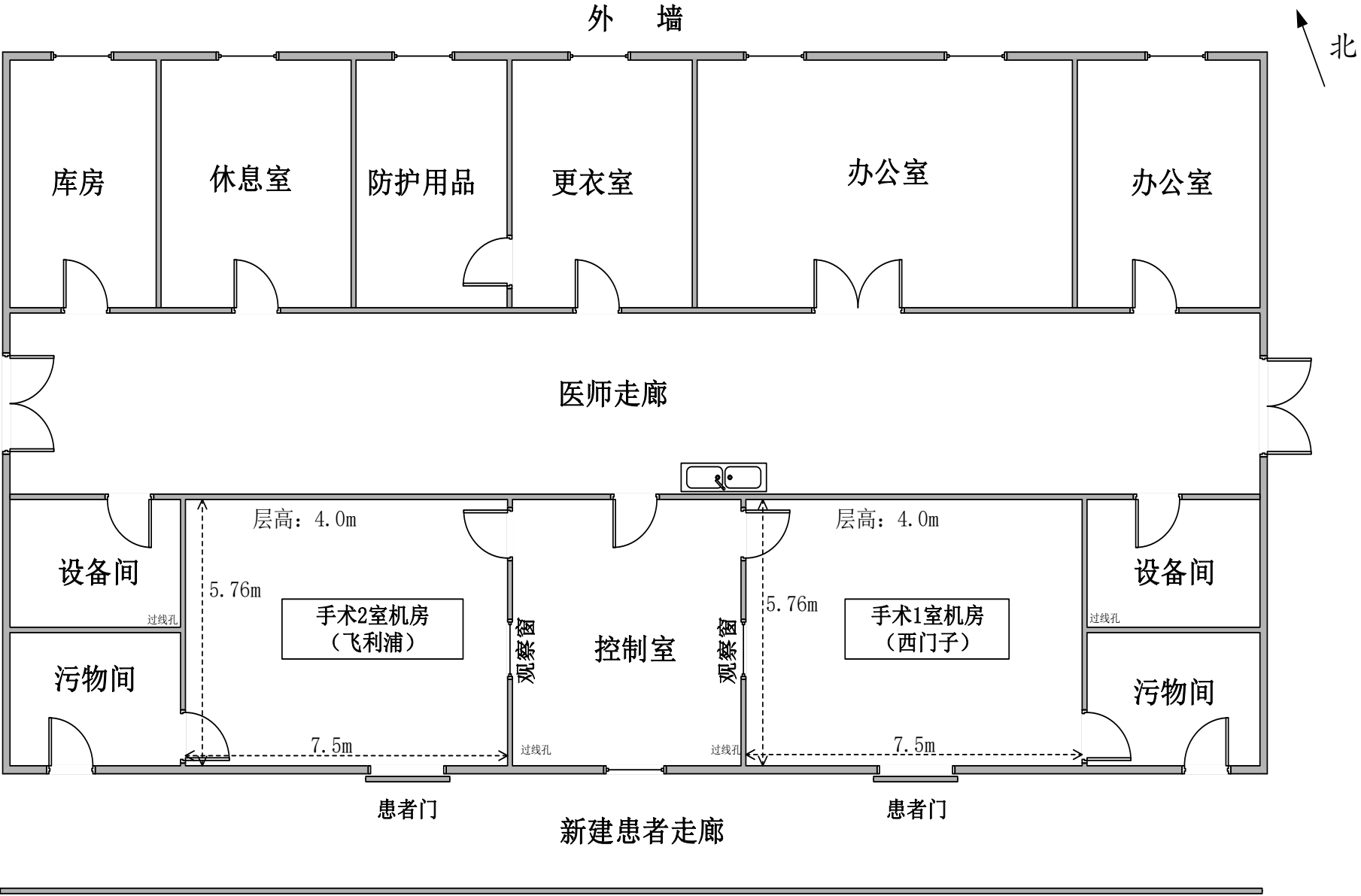
附图 3 大同三医院 DSA 工作场所平面图
