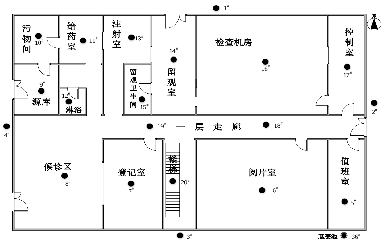
图 4.2 退役核医学科楼一层 \gamma 辐射剂量率的检测布点
