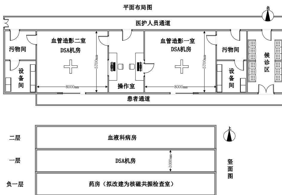
图 4.5 迁建 2 台 DSA 工作场所辐射剂量检测布点
