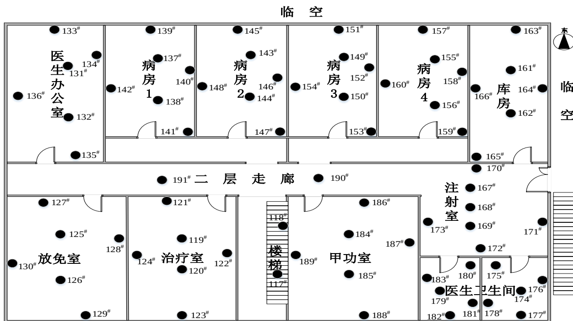
图 4.3 退役核医学科楼二层 \beta 表面污染的检测布点
